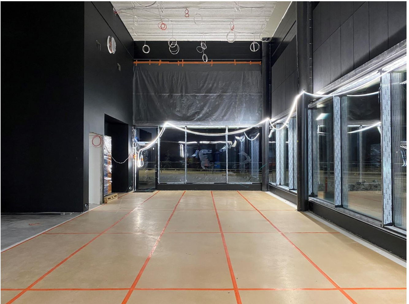
Kuva 1 R1 sisäänkäyntirakennuksen betonilattia hiottu, käsitelty ja suojattu. Myös akustointilevyjä asennettu seiniin.
